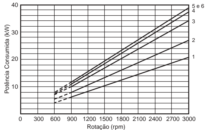
Curvas: Rotação x Potência
